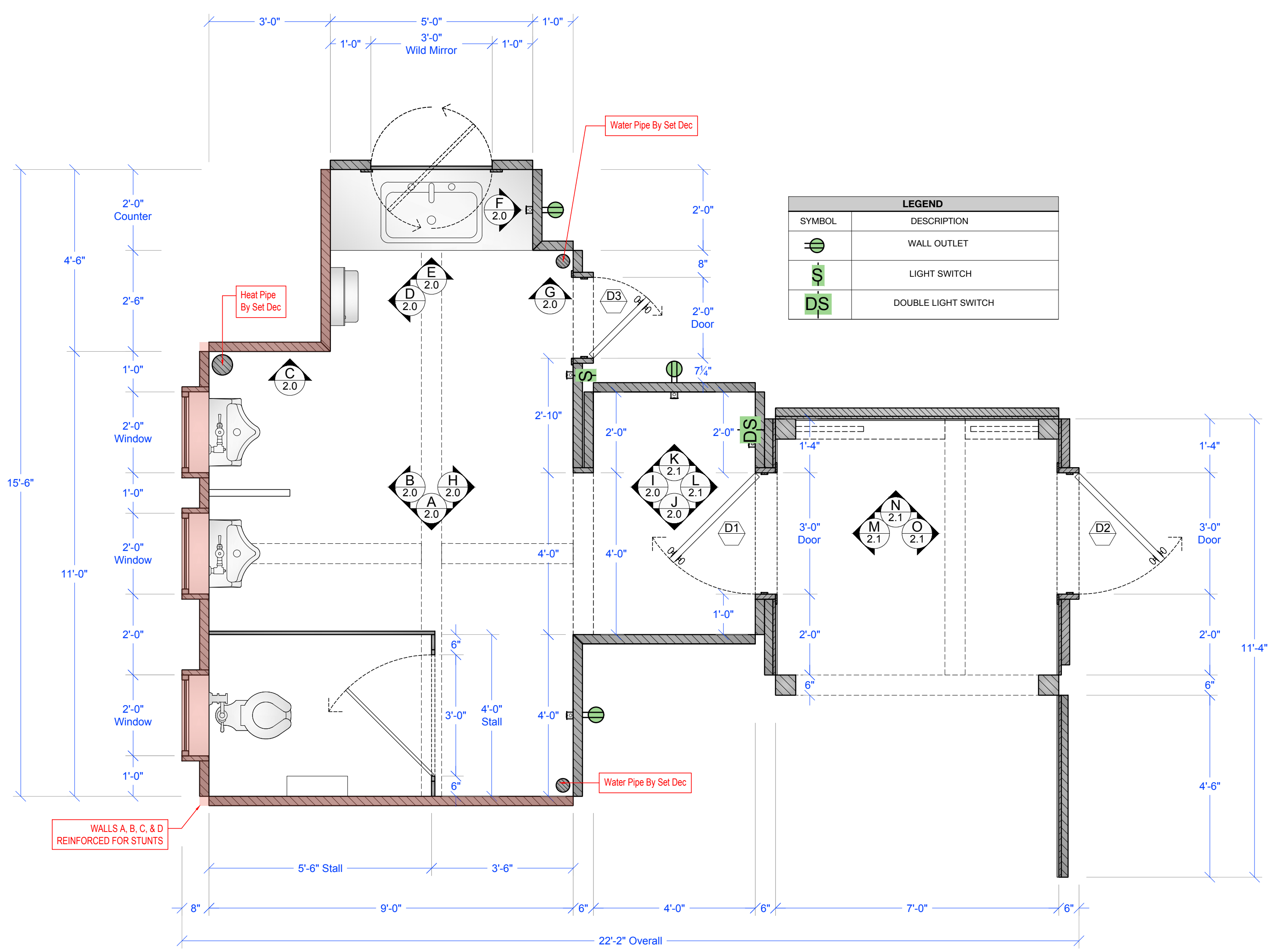
1 SET PLAN SCALE: 1/2" = 1'-0"
